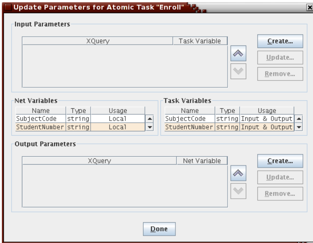
Fig. 31: Updating Parameters for a Task
