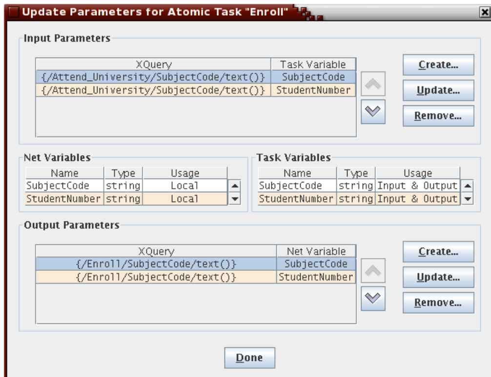
Fig. 33: Established task parameters
